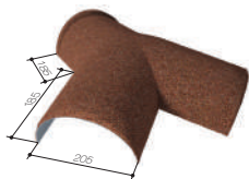
TRÓJNIK GĄSIORA 205 15-30°
