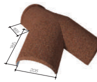
TRÓJNIK GĄSIORA 205 30-45°
