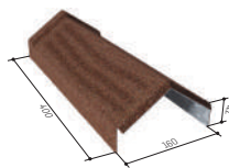
GĄSIOR CORONA/SENATOR
