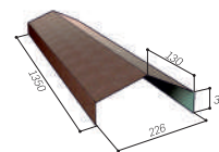
GĄSIOR DŁUGI CORONA AR130
