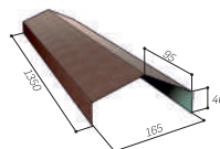
GĄSIOR DŁUGI CORONA AR95
